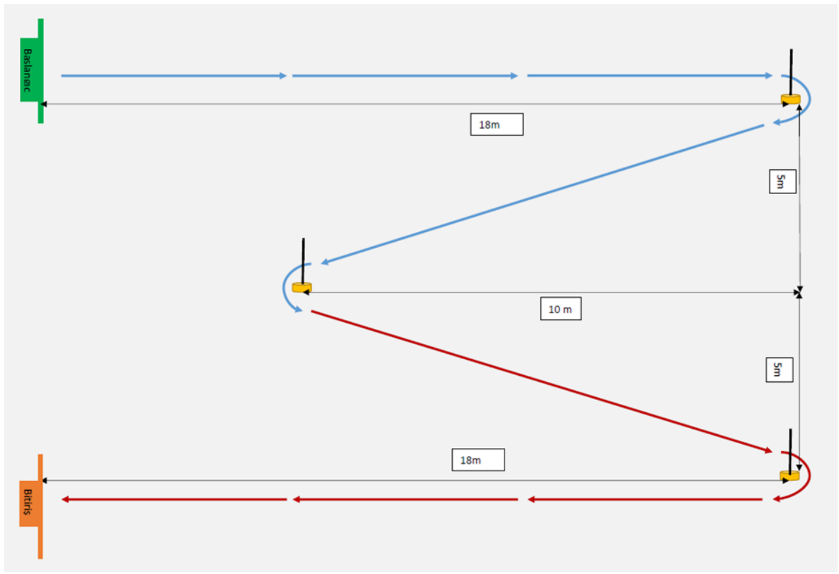
Şekil 5. Özel Gereksinimi Olan (Engelli) Aday Test Parkuru
